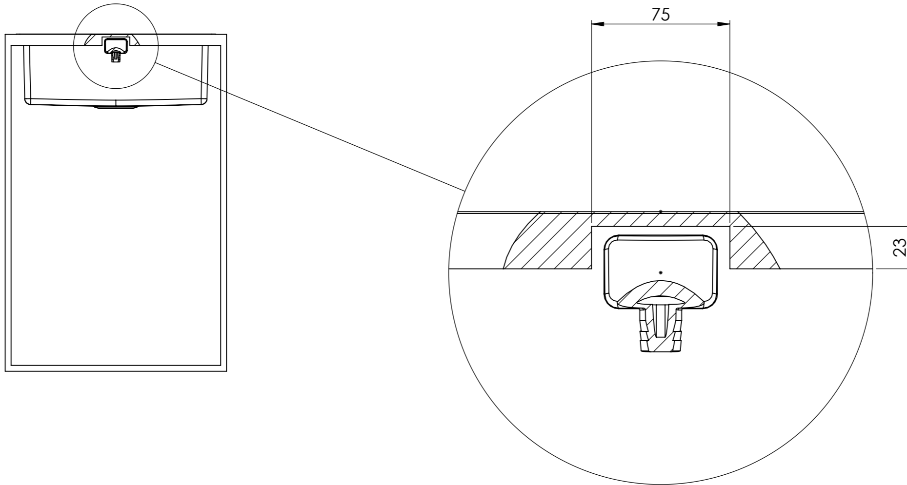
DETAIL AB SCALE 1 : 2
