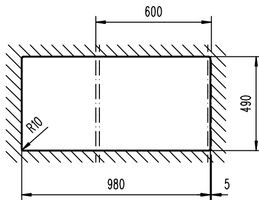
Ausschnitt übergreifend 1:20
